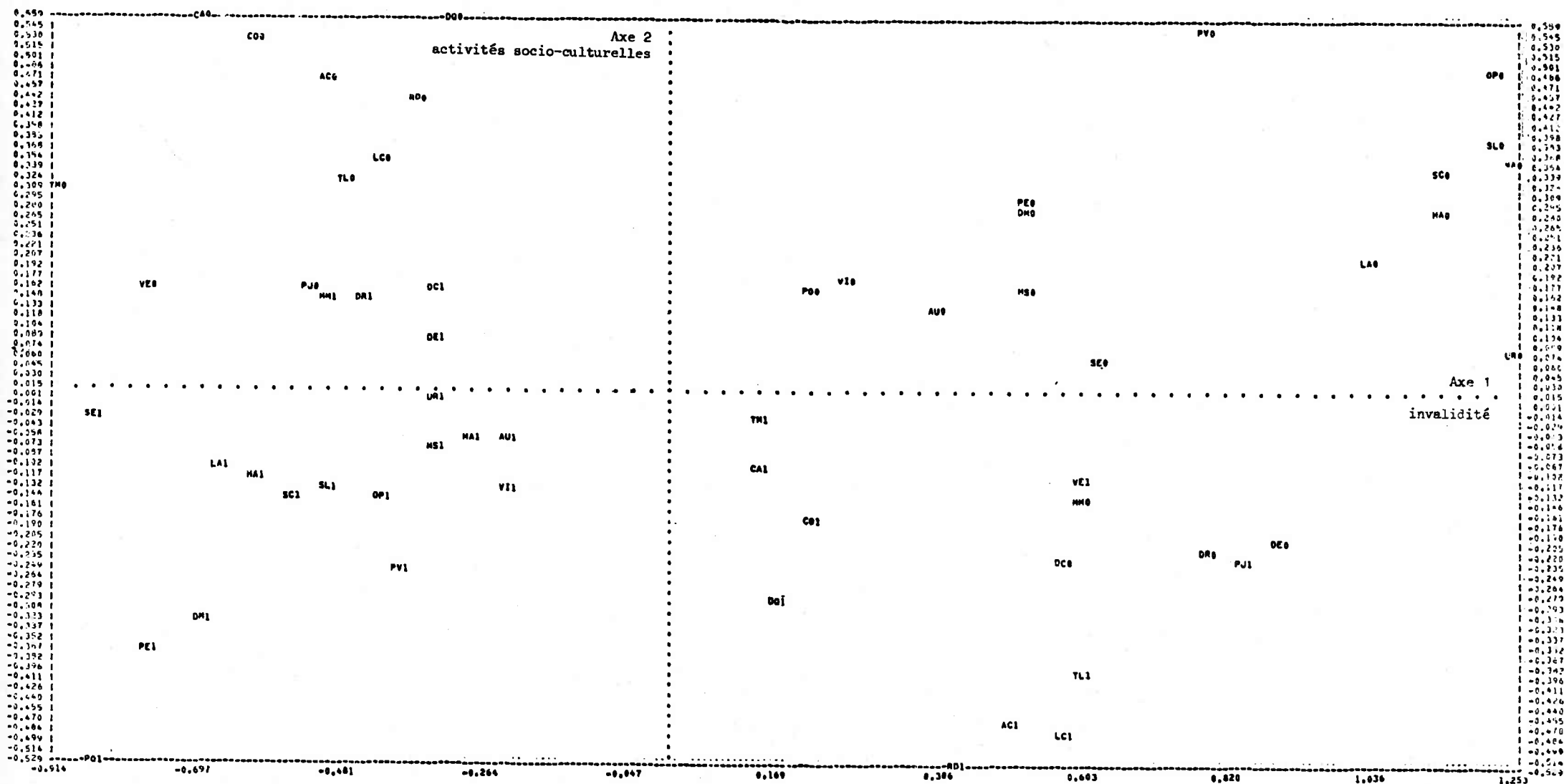
Graphique 12 : Analyse des correspondances . Projection des variables dans le plan des deux premiers axes (variables enregistrées en oui ou non)
