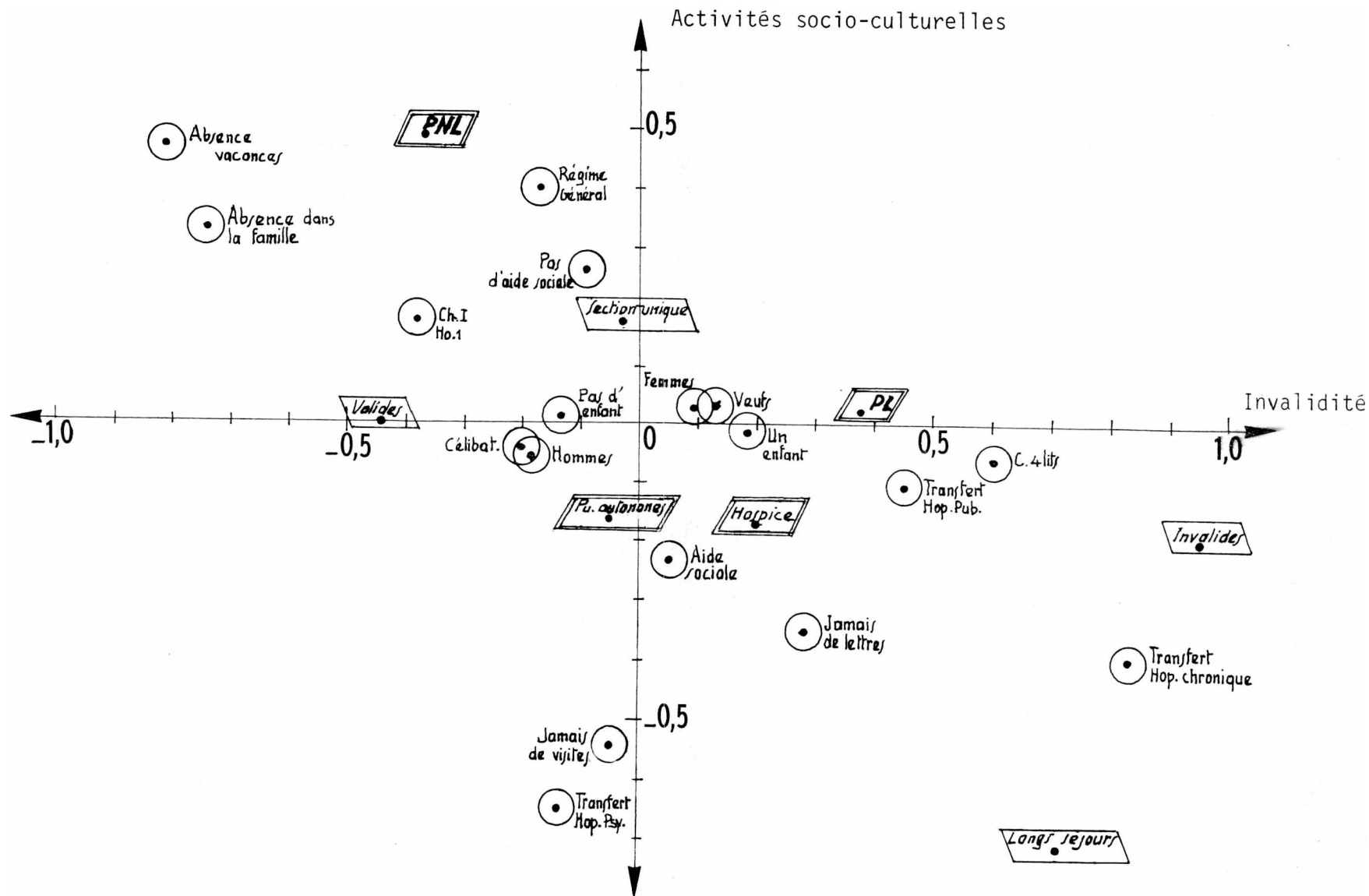
Graphique 13 : Projection des diverses variables dans le plan des deux premiers axes
